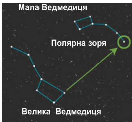
Мал. 63. Як знайти Полярну зорю
