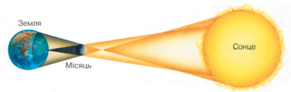
Мал. 100. Схема сонячного затемнення
