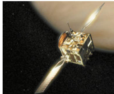
Мал. 84. Сучасна техніка для вивчення Всесвіту
