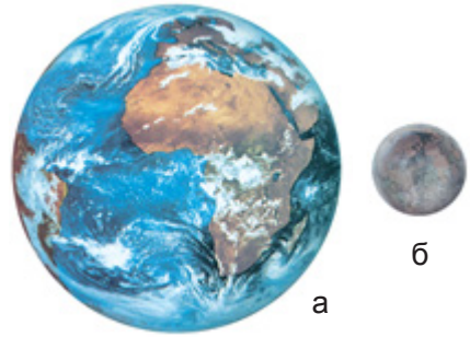
Мал. 97. Порівняльні розміри Землі (а) і Місяця (б)
