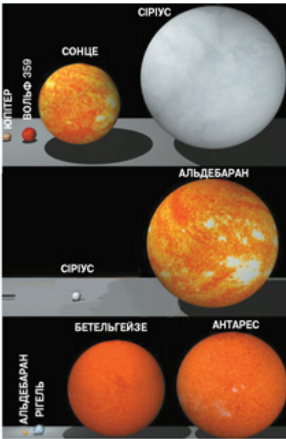
Мал. 64. Порівняльні розміри деяких зір
