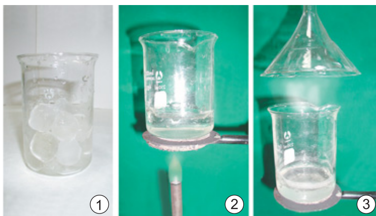
Мал. 18. Перехід води з одного агрегатного стану в інший
