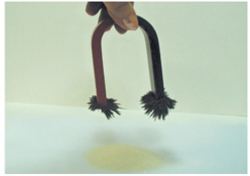
Мал. 29. Дослід з розділення суміші цукру і заліза
