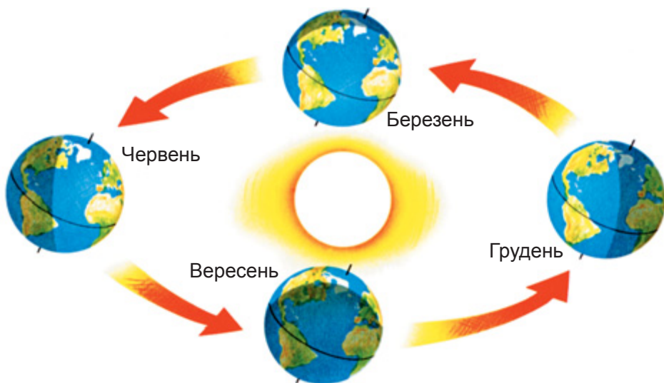
Мал. 96. Річний рух Землі навколо Сонця
