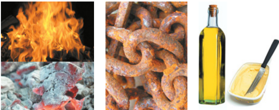
Мал. 35. Хімічні явища
