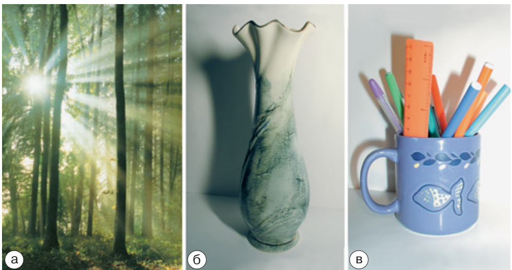
Мал. 49. Поширення світла (а) та утворення тіні (б, в)
