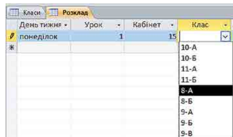
Мал. 3.17. Список підстановки в полі Клас таблиці Розклад
