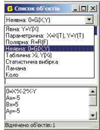
Мал. 2.36. Спадний список вікна Список об'єктів
