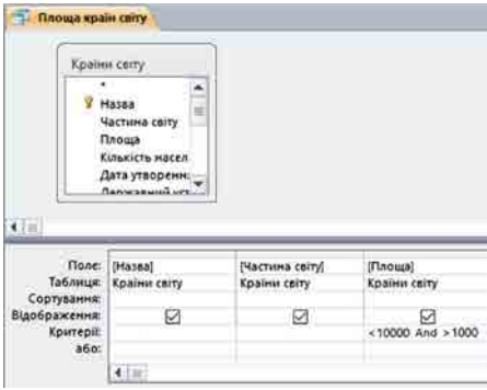
Мал. 3.40. Фрагмент вікна запити Площа країн світу у поданні Конструктор
