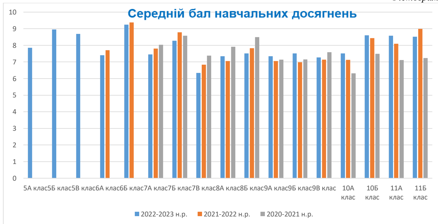
Гістограма 3
