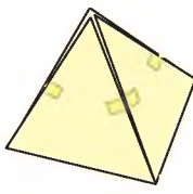
Складений тетраедр
