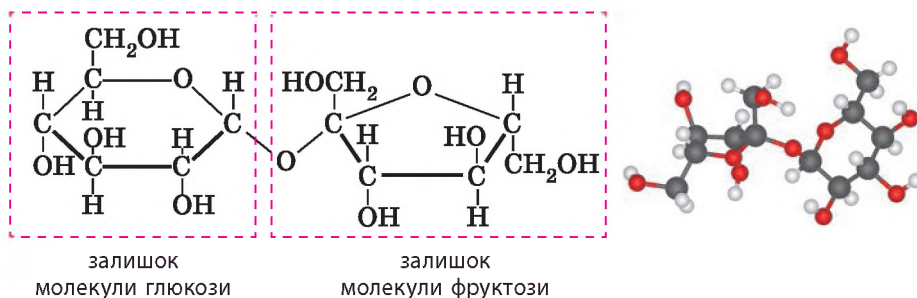
сахароза
