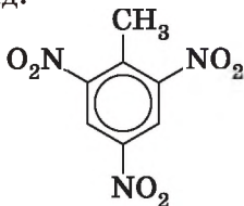
тринітролуен (тротил)
