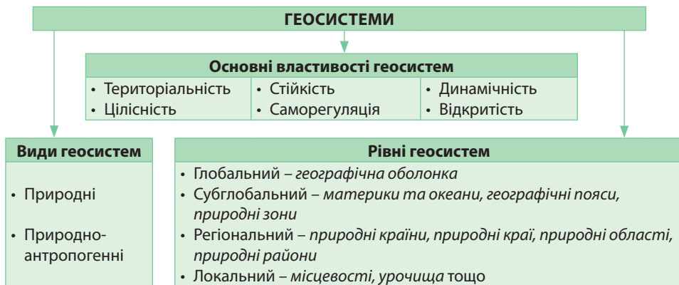
Мал. 2. Геосистеми
